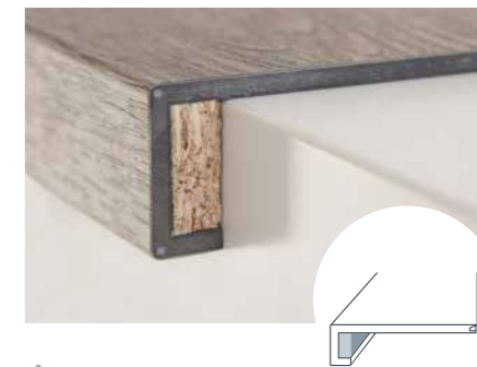
TYP C Doppelt gebogen, bis 5 mm Materialstärke – mit Einlage
