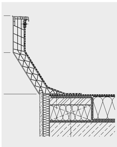
Eindichten Aufsetzkranz 3020
