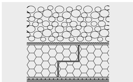
Umkehrdach
