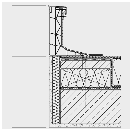
Eindichten Aufsetzkranz 1600
