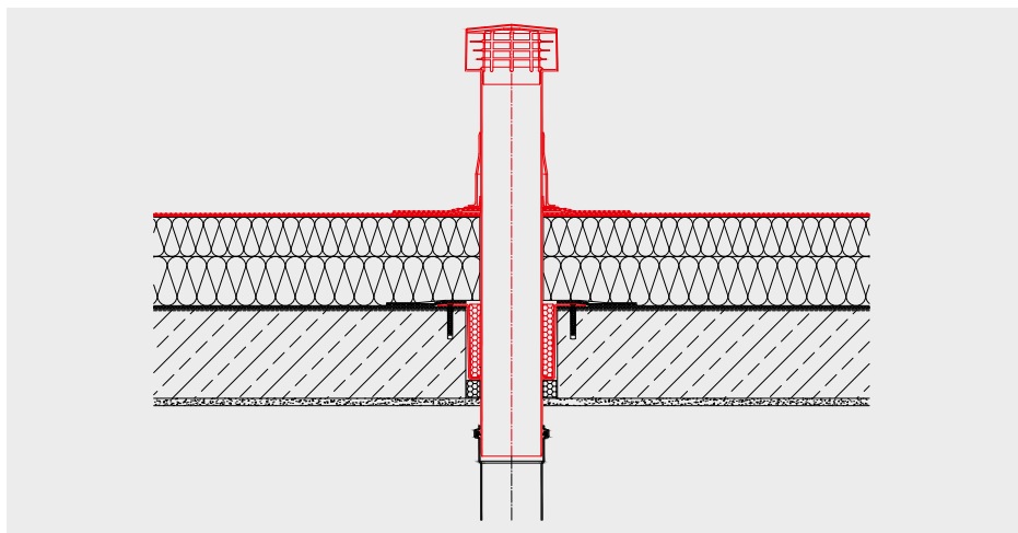
alwitra-Strangentlüfter (2-teilig)
