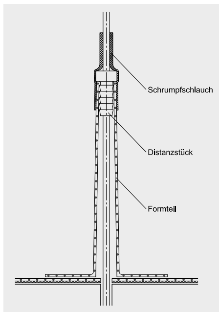
Durchdringungen Ø 8 - 10 mm
