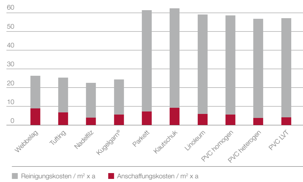
Jahreskosten verschiedener Bodenbelagsarten (CHF pro m 2 x a)
