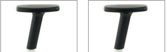
4D armrests no. 18, adjustable in height, width and depth, arm pad swings out. Accoudoirs 4D n° 18, réglables en hauteur, largeur et profondeur, manchette pivotante.
